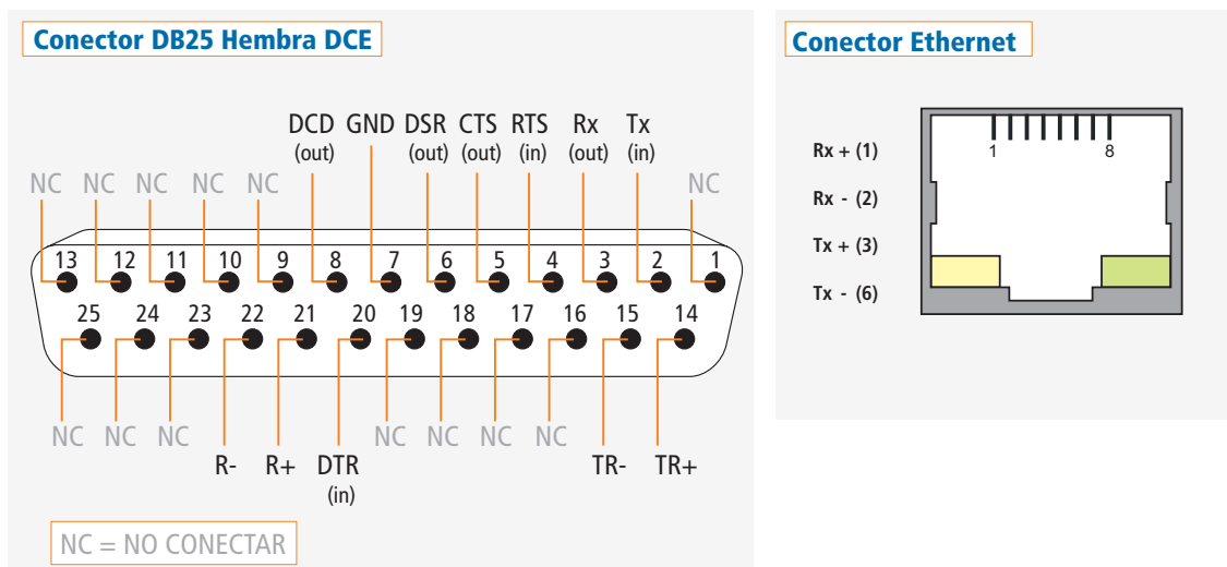
Figura 11 - Conectores
